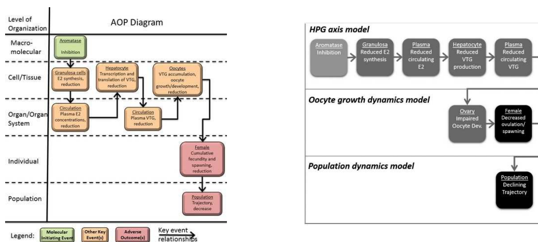
Figure 1. Schéma de l'AOP (à gauche ; Villeneuve, 2016) et de l'AOP quantitatif (à droite ; Conolly et al. 2017) de la perturbation du cytochrome P450 aromatase au niveau des gonades chez le fathead minnows.
